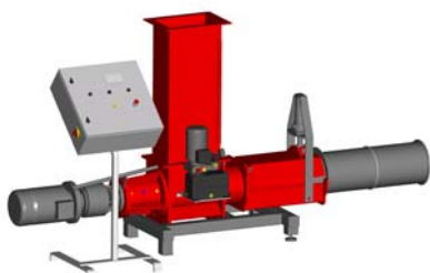
09-50115 SK240 til komprimering af brugte (næsten tomme) flasker
